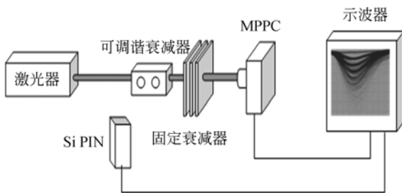
图 4 MPPC 光子探测实验装置实验图
