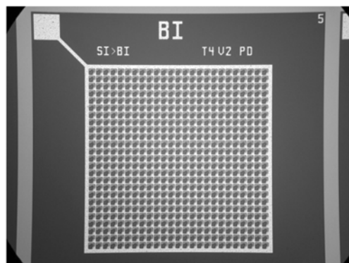
Fig. 1 Photo of MPPC module
