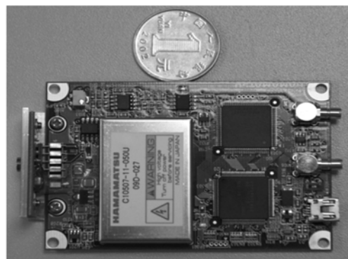
图1 MPPC模块实物图
